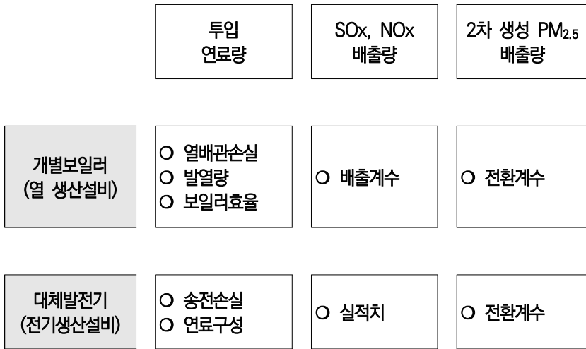
〈그림 2〉 대체설비의 대기오염물질 배출량 산정시 주요 고려사항
